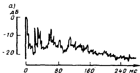
Рис. 6.23. Осциллограммы, снятые в партере универсального зала в Гаване
