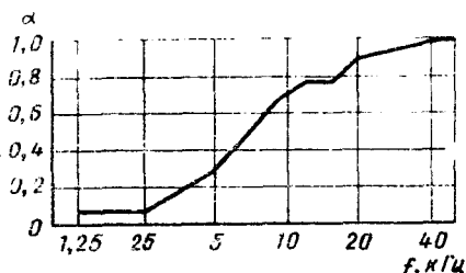
Рис. 4.4. Частотная характеристика коэффициента звукопоглощения \alpha слоя поролона толщиной 3 мм
