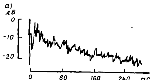
Рис. 6.24. Осциллограммы, снятые на балконе универсального зала в Гаване
