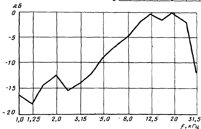
Рис. 4.9. Спектр искрового импульса
