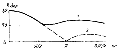
Рис. 1.13. Зависимость |R_K|_{cp} от расстояния между точками измерений 1 — свободное поле; 2 — диффузное поле
