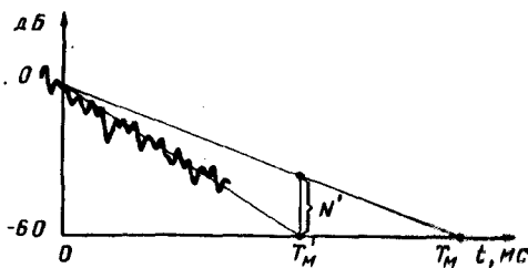
Рис. 4.19. Поправка на затухание звука в воздухе модели на высоких частотах в зависимости от времени пробега звуковой волны и частоты
