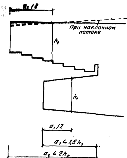
Рис. 5.2. Пазухи над и под балконом
